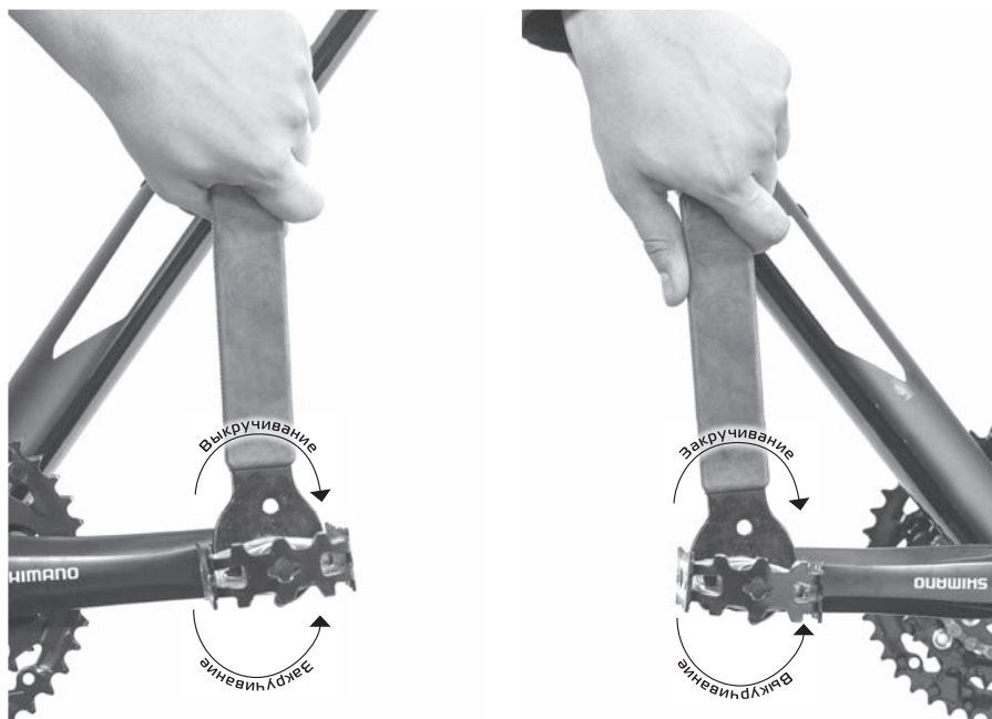
Рисунок 22. Направление вращения оси педалей. Фото слева — правая pedal. Фото справа — левая pedal
