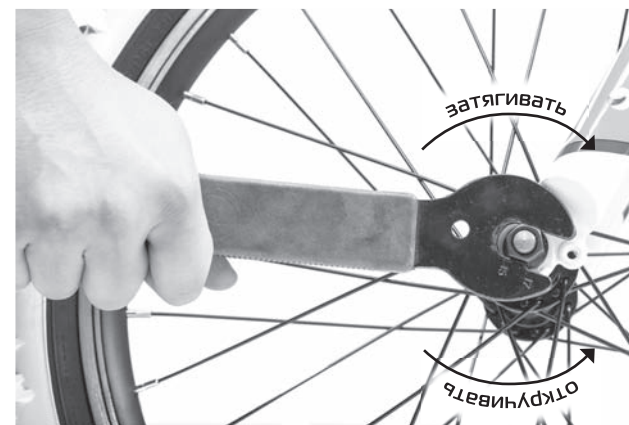
Рисунок 10. Затяжка гаек колесных осей происходит обычным образом: гайки затягиваются по часовой стрелке
