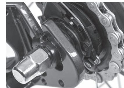
Рисунок 25. Регулировка натяжения тросика планетарной втулки
